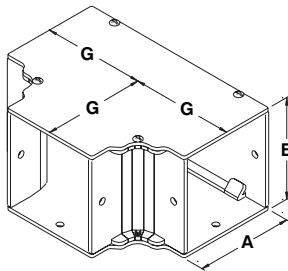
Raccord en 'T'
