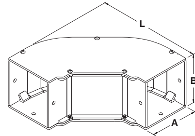
Coude à portée 90 degrés
