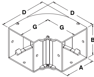
Coude 90 degrés
